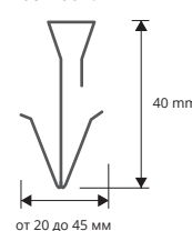
СРФХАС 40 масштаб 1:2
