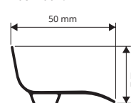
РЕТФХАА 50 масштаб 1:2
