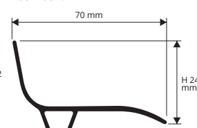
РЕТФХАА 70 масштаб 1:2
