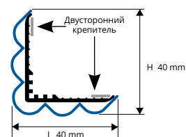
PFC... 40/40A масштаб 1:2
